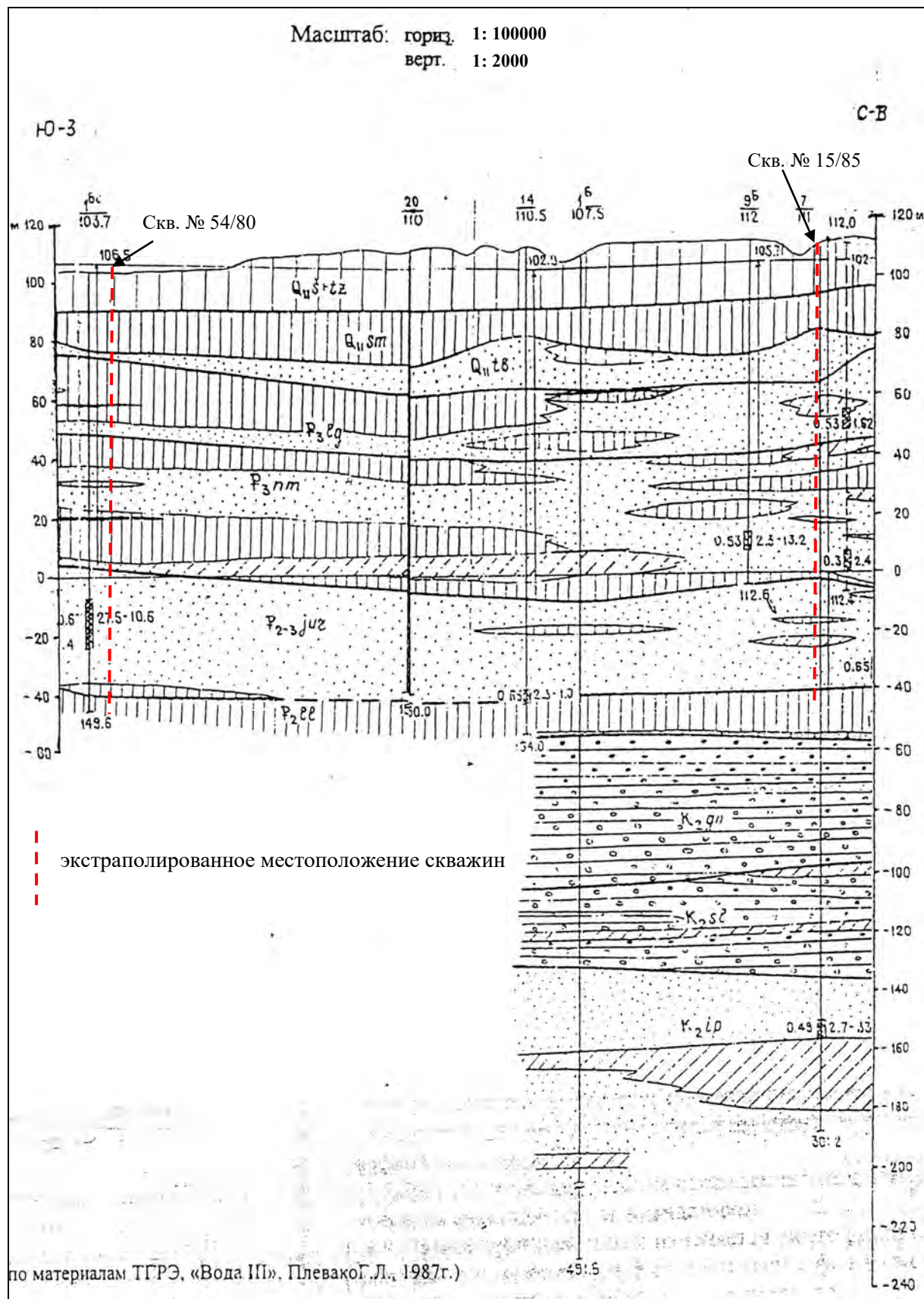
Рис 3. Региональный гидрогеологический разрез
